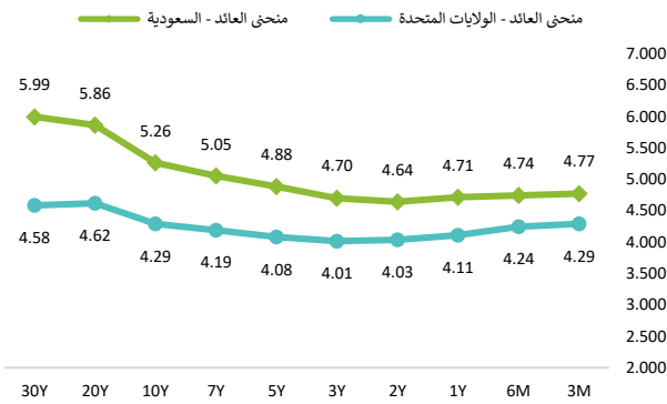
مقارنة منحنى العائد بين السعودية والولايات المتحدة
